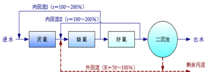
图 3.4-3 UCT 工艺流程图
