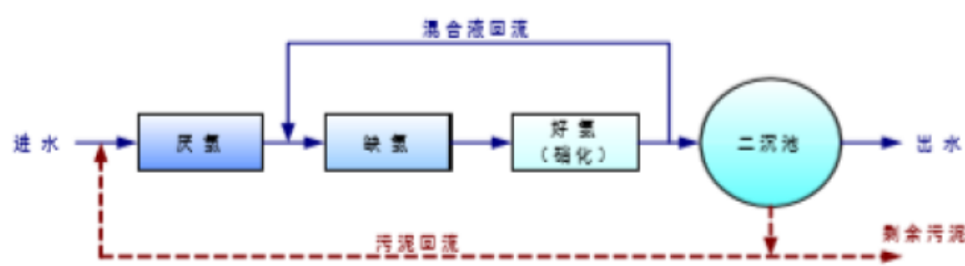
图 3.4-1 AAO 工艺流程图
