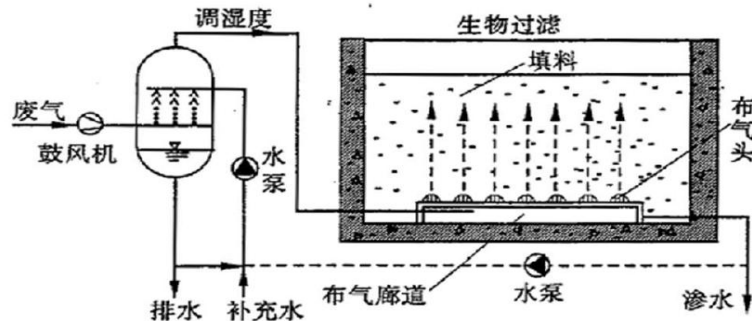
图 3.4-7 臭气处理工艺流程图
