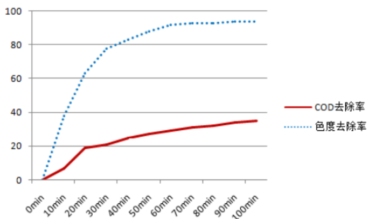
图 3.4-6 臭氧对 COD、色度去除率影响
