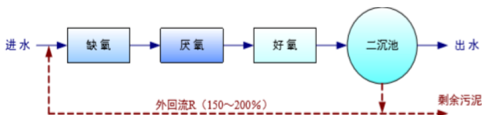
图 3.4-2 倒置 AAO 工艺流程图
