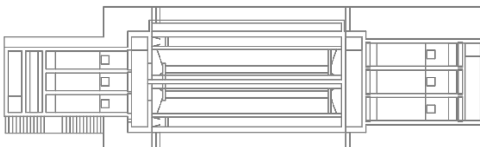
图 3.4-1 预处理工艺平面布置示意图
