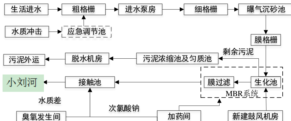
图 3.7-1 项目工艺流程图
