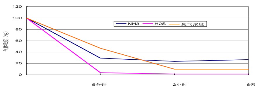
图 3.4-8 恶臭污染物转化过程示意图
