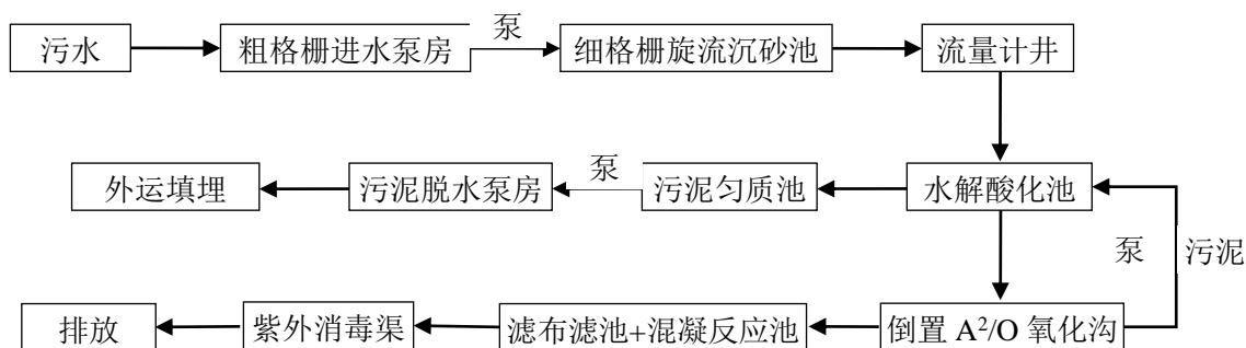
图 7-1 金风环保（沭阳）有限公司（原沭阳凌志水务有限公司）工艺流程图
